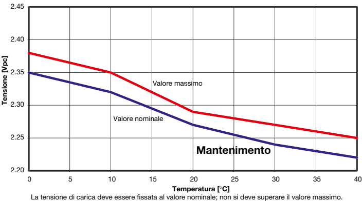
Fig. 1: Marathon L/XL e Powerfit S100/SL100/S300; tensione di carica vs. temperatura
