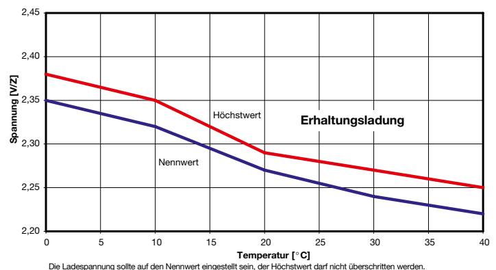
Bild 1: Marathon L/XL und Powerfit S100/S100L/S300; Ladespannung über der Temperatur
