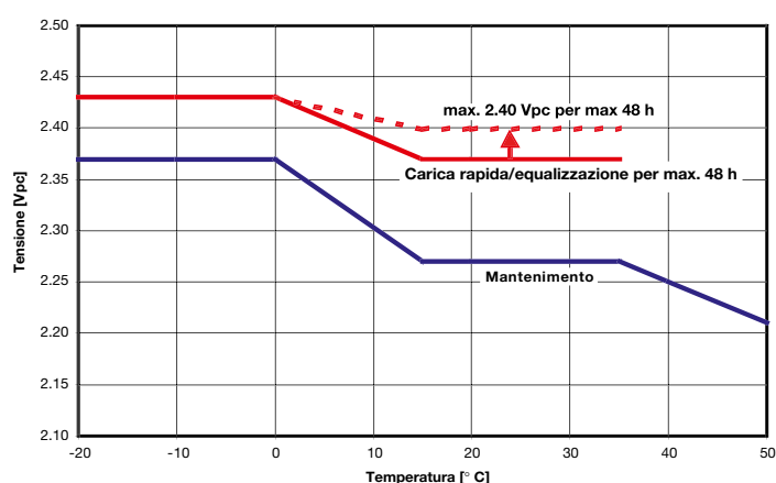
Fig. 3: A400/FT, A600, A700, Powercycle; tensione di carica vs. temperatura
