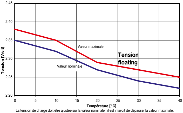
Figure 1: Marathon L/XL et Powerfit S100/S100L/S300; tension de charge en fonction de la température
