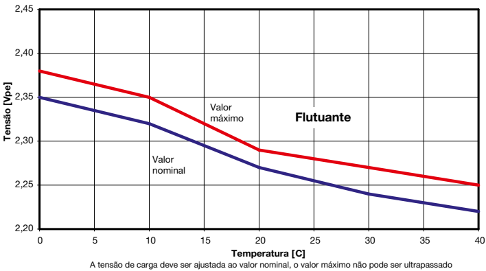
Fig.1: Marathon L/XL e Powerfit S100/SL100/S300; Tensão de carga vs. Temperatura
