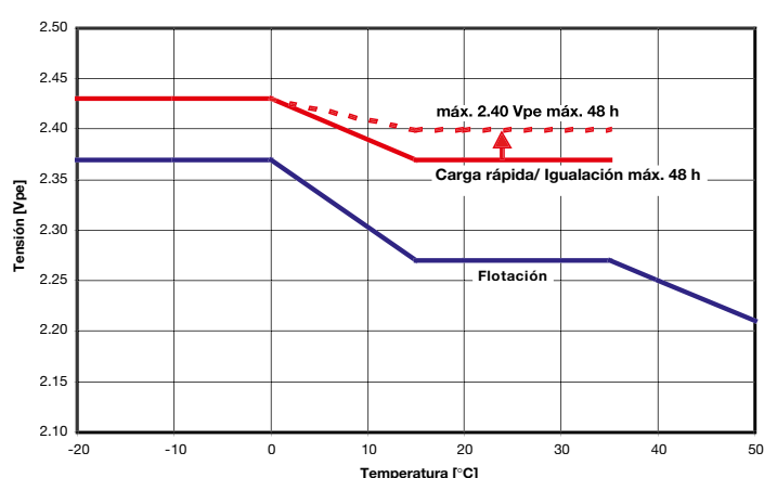
Fig. 3: A400/FT, A600, A700, Powercycle; tensión de carga vs. temperatura
