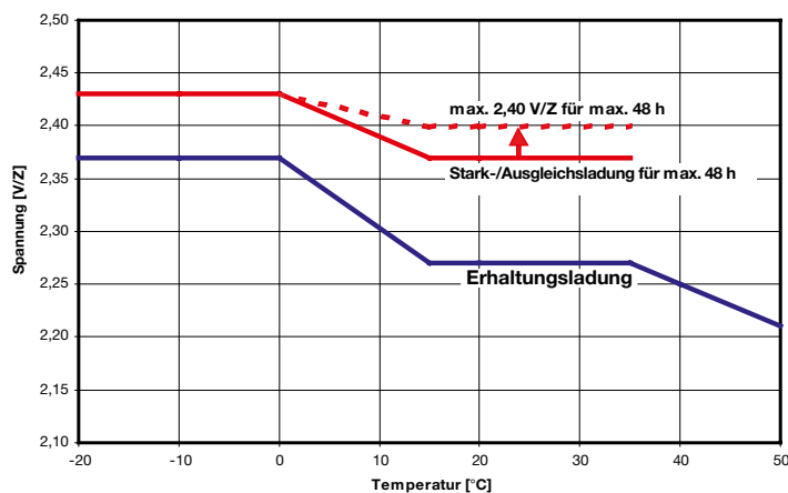
Bild 3: A400/FT, A600, A700, Powercycle; Ladespannung über der Temperatur
