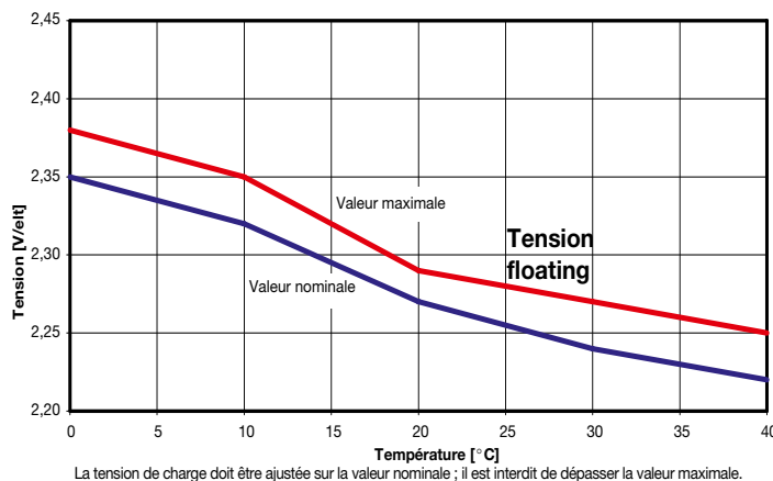
Figure 1: Marathon L/XL et Powerfit S100/S100L/S300; tension de charge en fonction de la température
