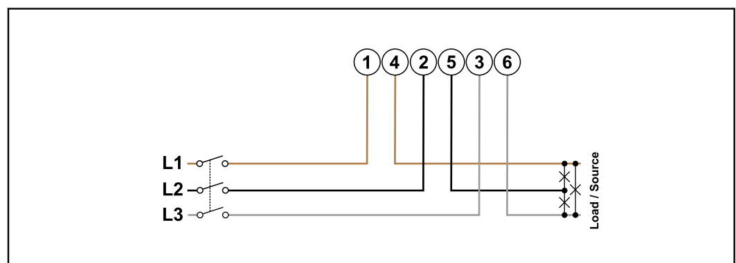
3 Phasen, 3 Leiter
