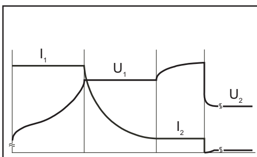
„Refresh“-Kennlinie IUIoU:
