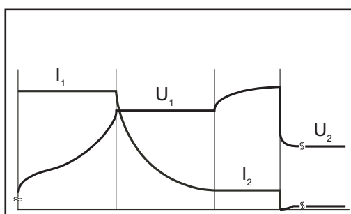
Curva característica de "Atualização" IUloU:
