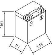
Maße
