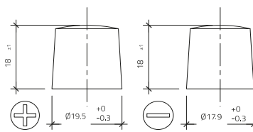
Polausführung 1
