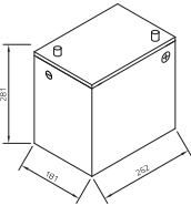
Maße
