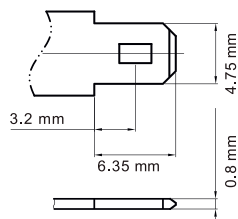
Polausführung S-4.8
