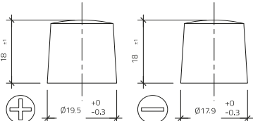
Polausführung 1
