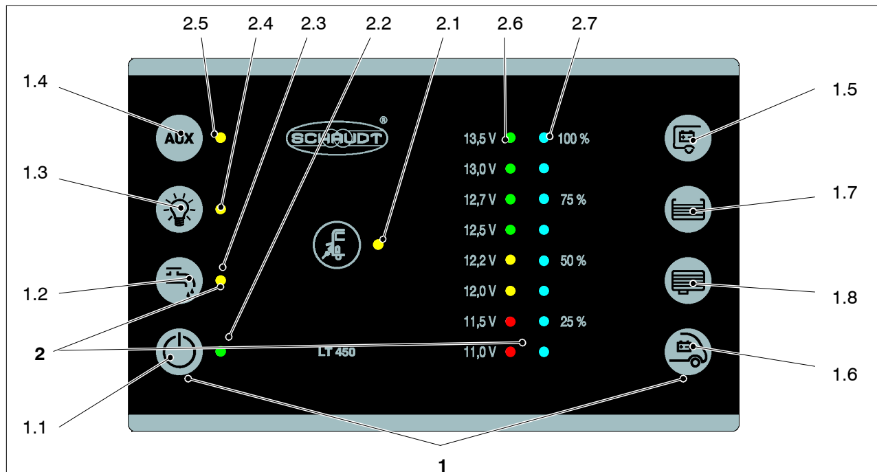
Bild 2 Aufbau Bedien- und Kontrollpanel LT 45X
