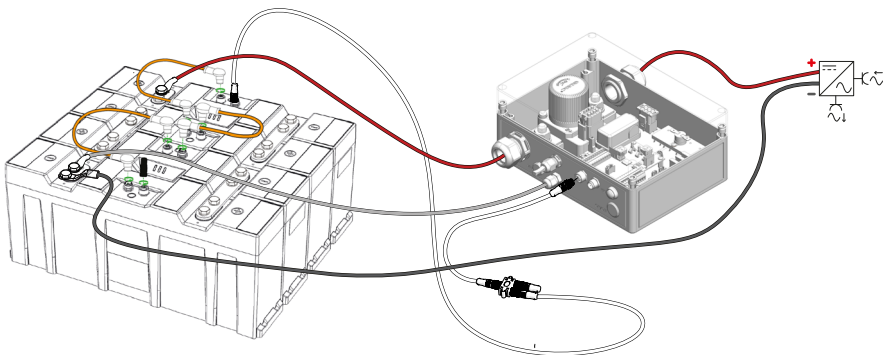
Abbildung 5. Anschluss einer Li-Ionen-Batterie an die SB-BIB
