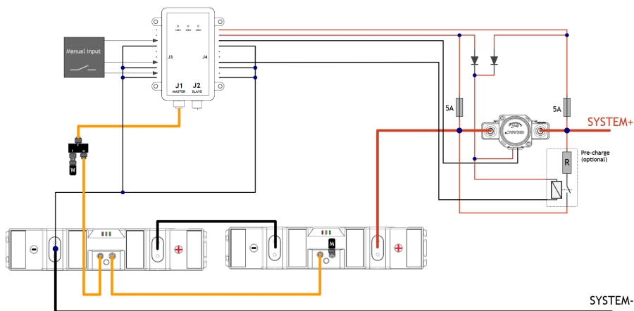
Abbildung 6. Anschluss einer Li-Ionen-Batterie an die BCI
