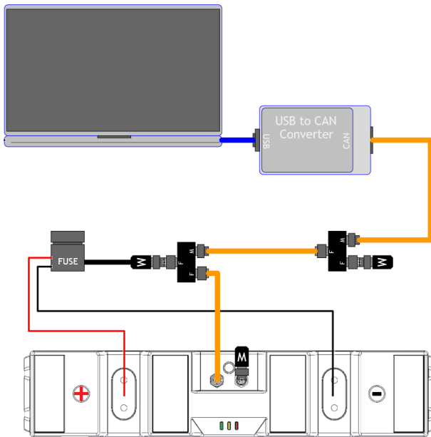
Abbildung 10. CAN-Bus-Stromversorgung
