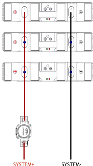
Abbildung 8. Drei Li-Ionen-Batterien parallel zur externen Abschaltvorrichtung
