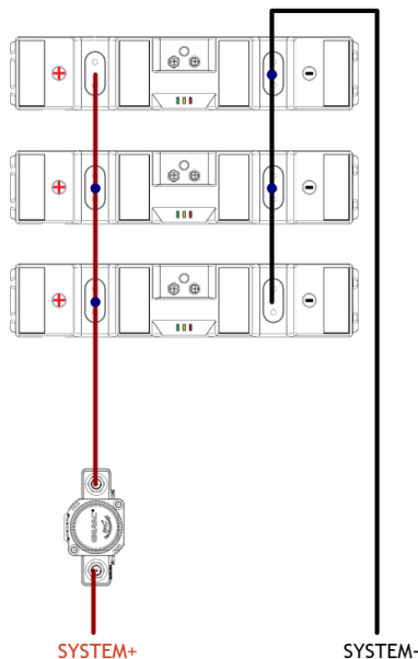
Abbildung 8. Drei Li-Ionen-Batterien parallel zur externen Abschaltvorrichtung
