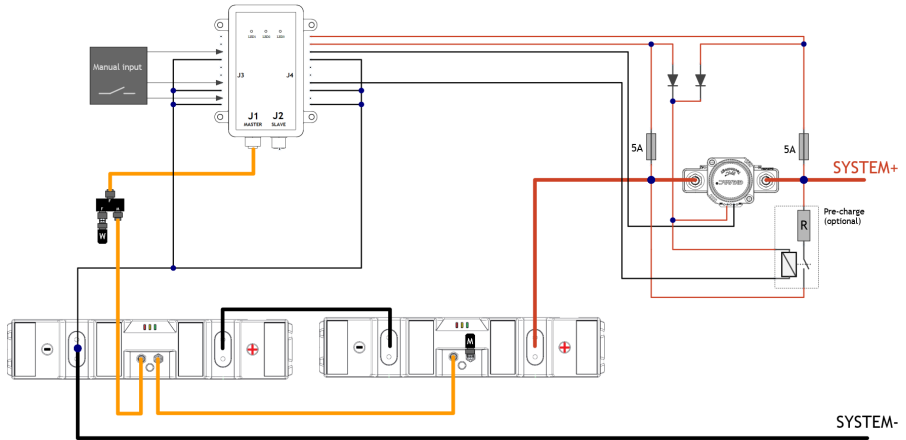
Abbildung 7. Die Batterien sind mit einer externen Abschaltvorrichtung und einer BCI in Reihe zu schalten.
