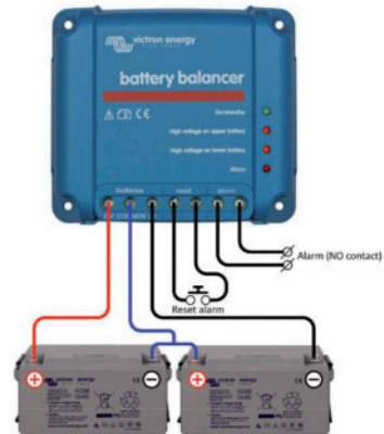
Battery Balancer (BMS012201000) Der Battery Balancer (Ladungszustandsausgleicher) gleicht den Ladezustand von zwei in Serie geschalteten 12 V Batterien oder von mehreren parallelen Strängen von in Serie geschalteten Batterien aus. Wenn die Ladespannung eines 24 V-Batteriesystems auf über 27 V ansteigt, schaltet sich der Battery Balancer ein und vergleicht die Spannung bei den zwei in Serie geschalteten Batterien. Der Battery Balancer entnimmt der Batterie (oder den parallel geschalteten Batterien) mit der höchsten Spannung einen Strom von bis zu 1 A. Der daraus resultierende Unterschied beim Ladestrom sorgt dann dafür, dass sich alle Batterien an denselben Ladezustand angleichen. Falls notwendig können mehrere Balancer parallel geschaltet werden. Eine 48 V Batterie-Bank kann mit drei Battery Balancern ausgeglichen werden.
